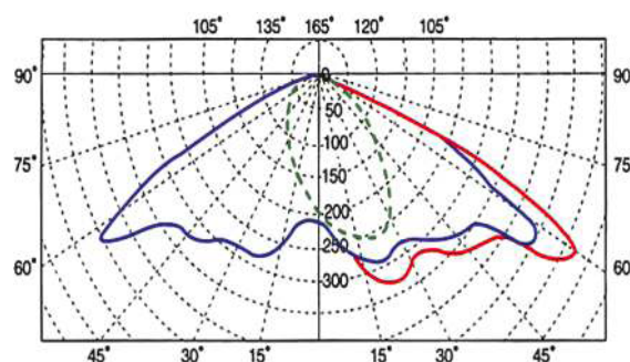
Křivka svítivosti
